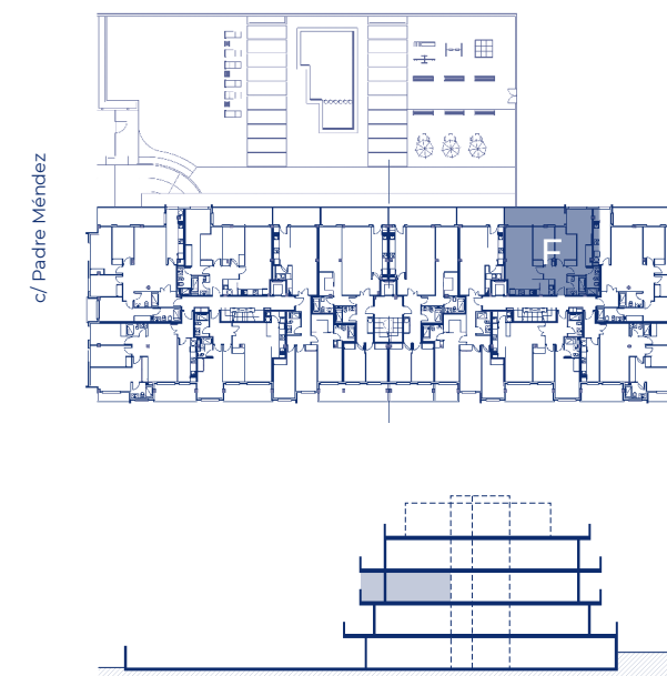
PLANTA 1
